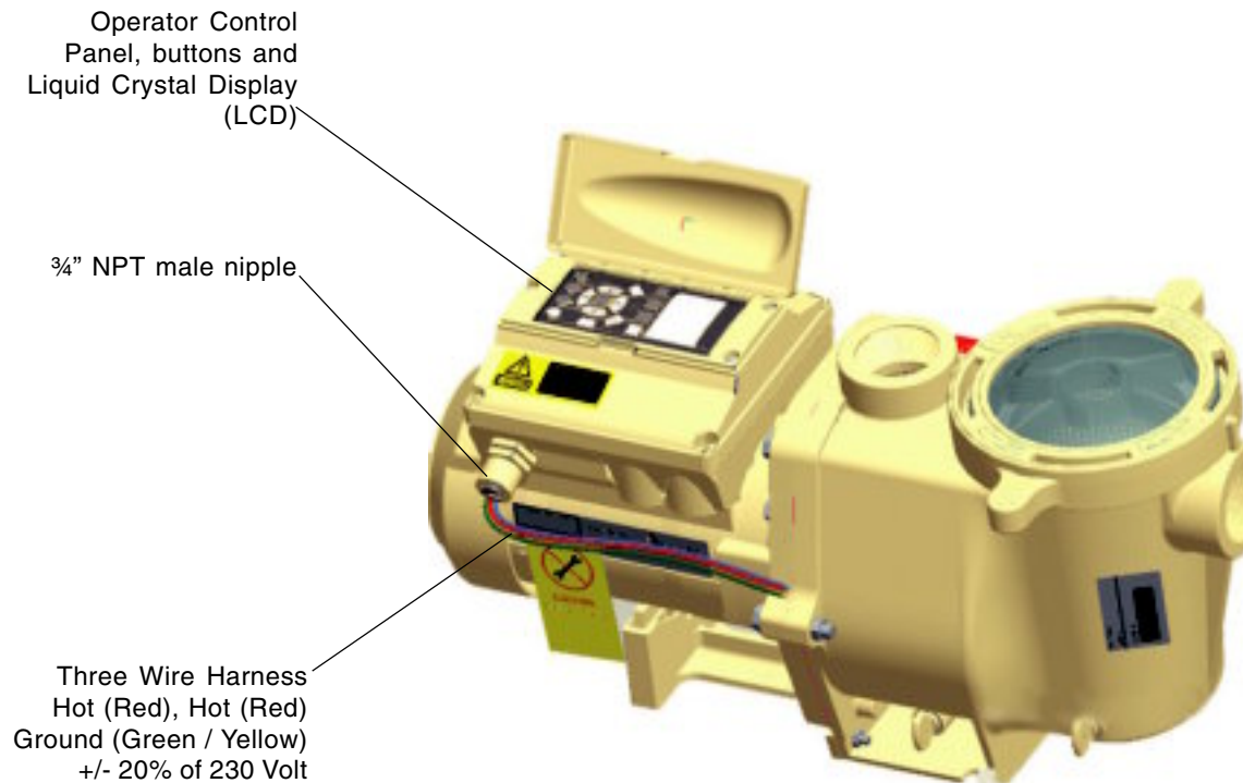
IntelliFlo VF Drive Assembly
